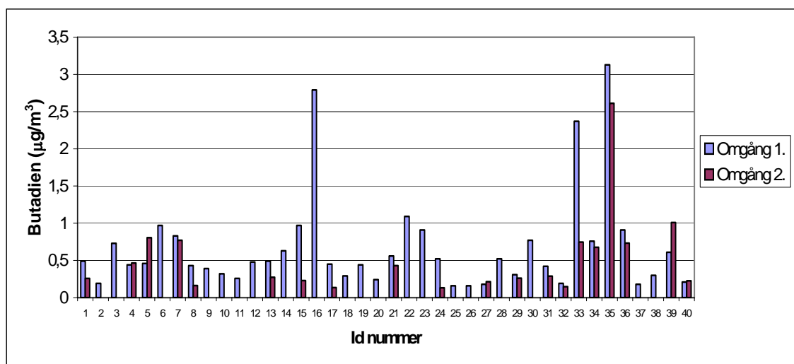
Figur 3. 1,3-Butadienkoncentrationen vid personburen mätning. Omgång 2 avser de 20 försökspersoner på vilka mätningarna upprepades.
